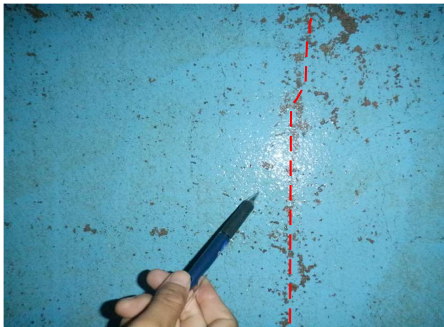
배수지2지 벽체 균열(0.3mm미만)
